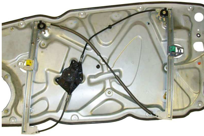
POWER WINDOW LEFT ALZACRISTALLI ELETTRICO SX
